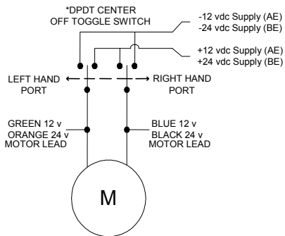
Wiring Diagram: AE & BE
